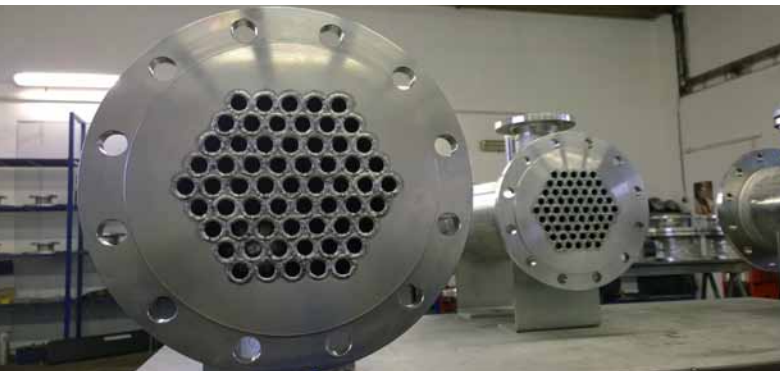
Trubkové výměníky tepla
